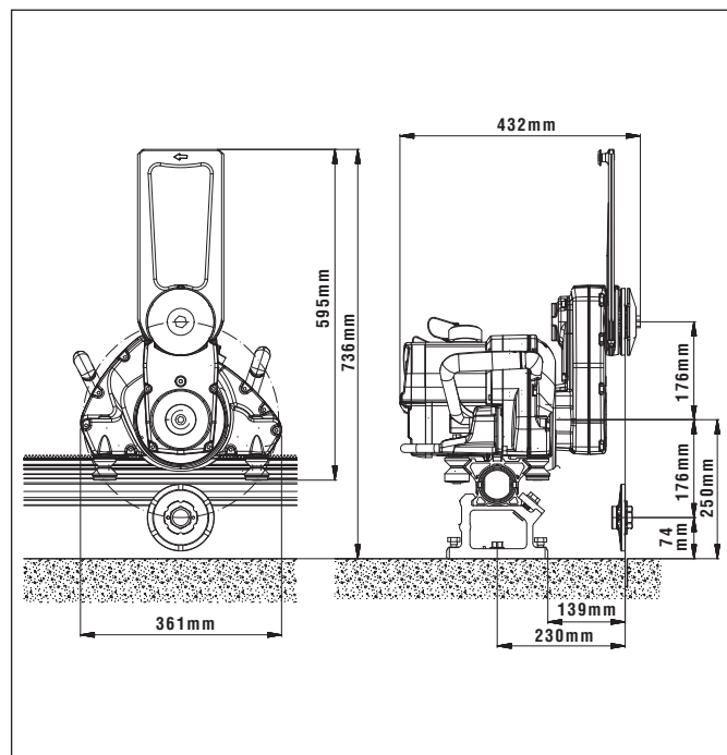
DS TS20-E sähköseinäsahan päämitat (mm)
