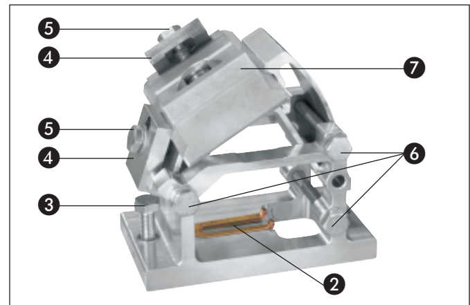
Kiskopukki kulma- ja porrassahauksiin
